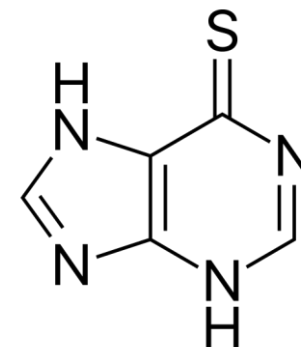
Mercaptopurine
